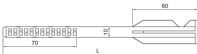
PREDNÝ POHĽAD
