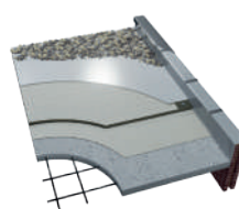
voľné polozenie fólie so záťažovou vrstvou
